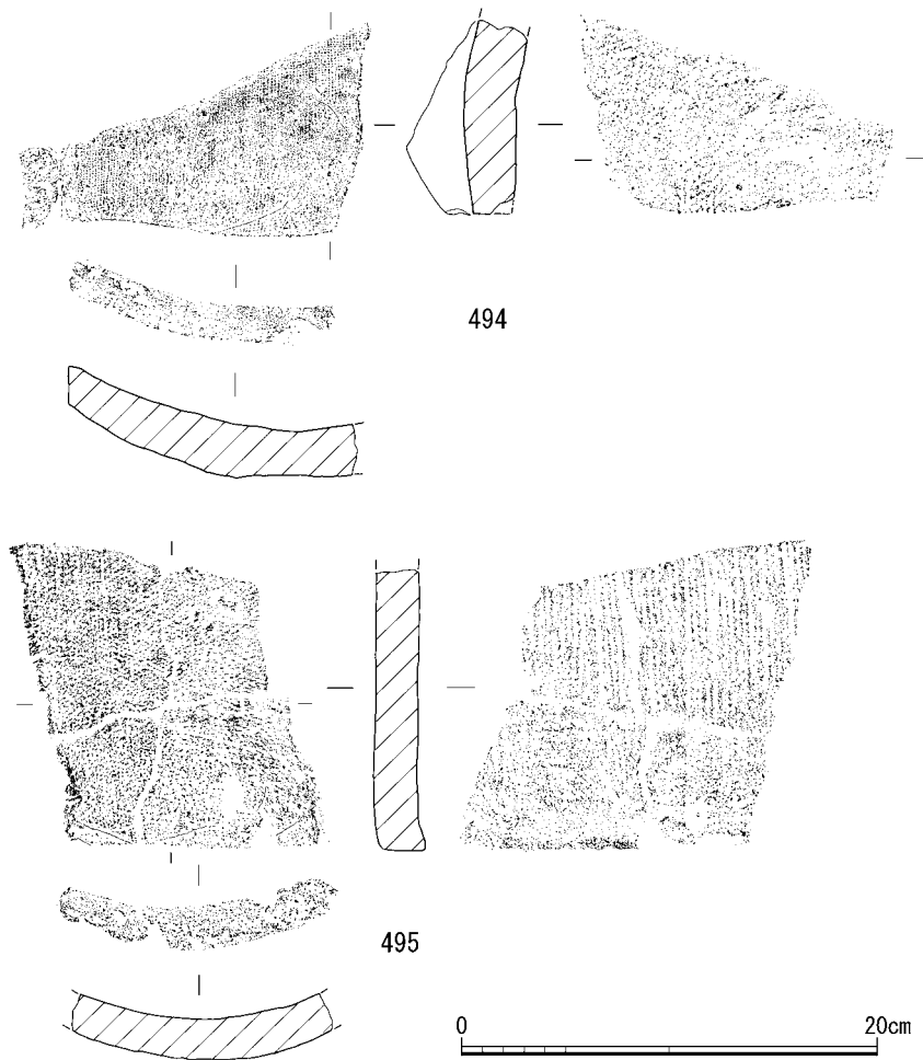
第111図 瓦実測図(3)
