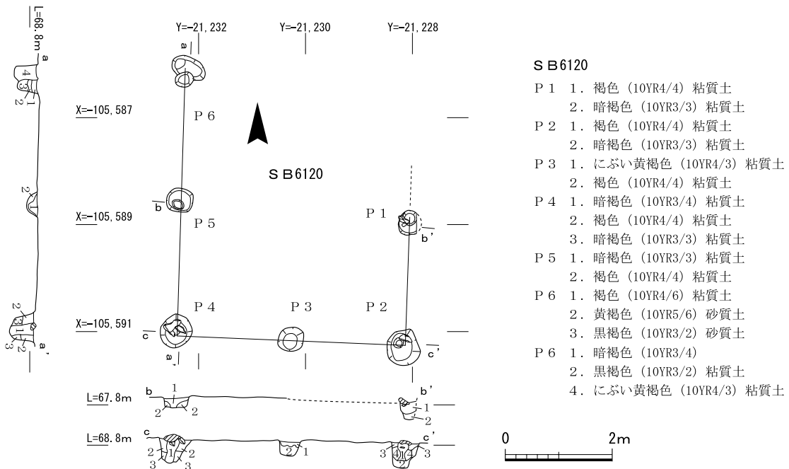
第61図 6区掘立柱建物 S B 6087・6120平面・断面図
