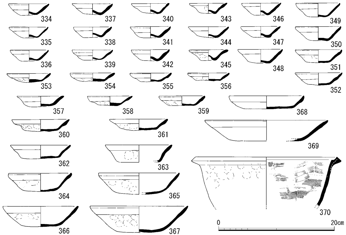
第55図 出土遺物実測図 S K 125・251
