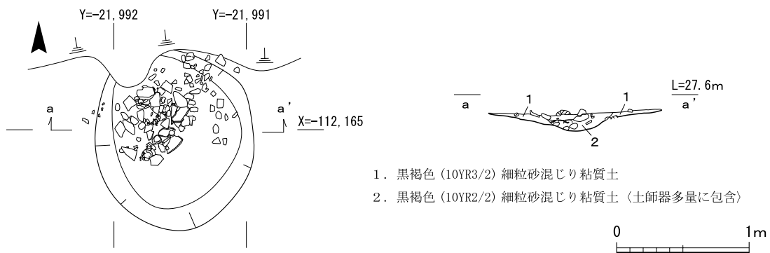
第36図 S K 287・288実測図
