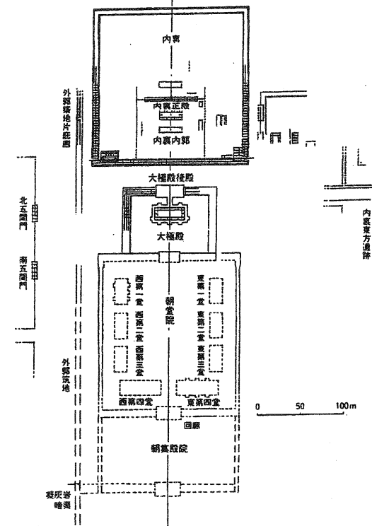
27 後期難波宮遺構配置図 (中尾芳治作図)
