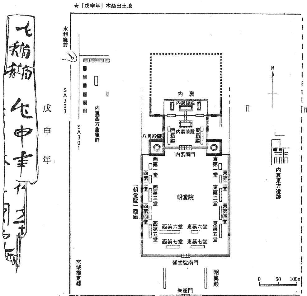
26 前期難波宮遺構配置図 (『難波宮址の研究』第11に加筆)
