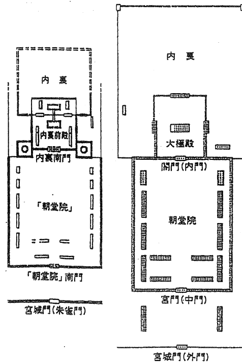
20 前期難波宮(左)、藤原宮(右) 内裏・朝堂院比較図
