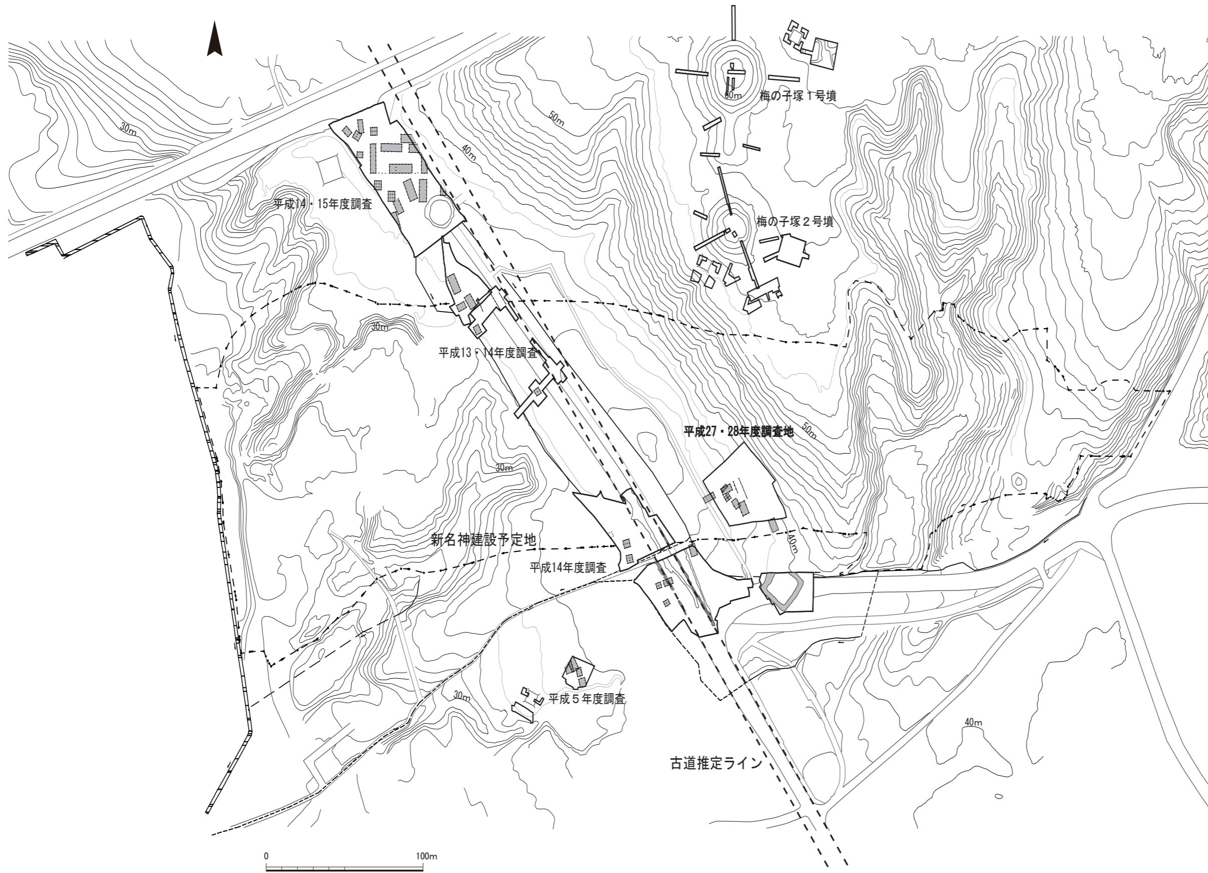
第3図 芝山遺跡 遺構配置図
